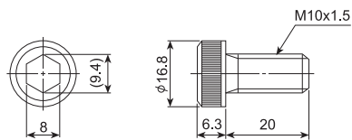
附固定專用螺栓 (M10X20特殊扁頭型內六角沈頭螺栓)
