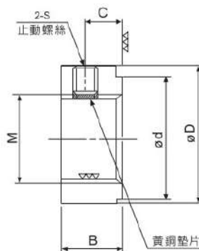
X-X剖面
